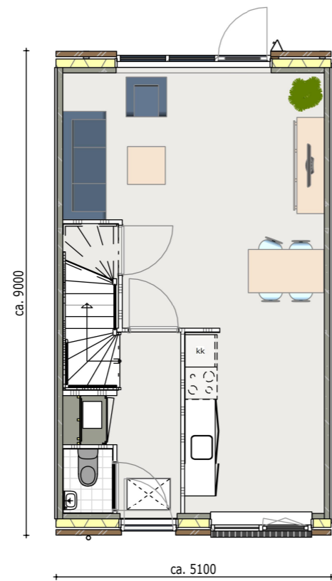
voorlopig ontwerp begane grond
